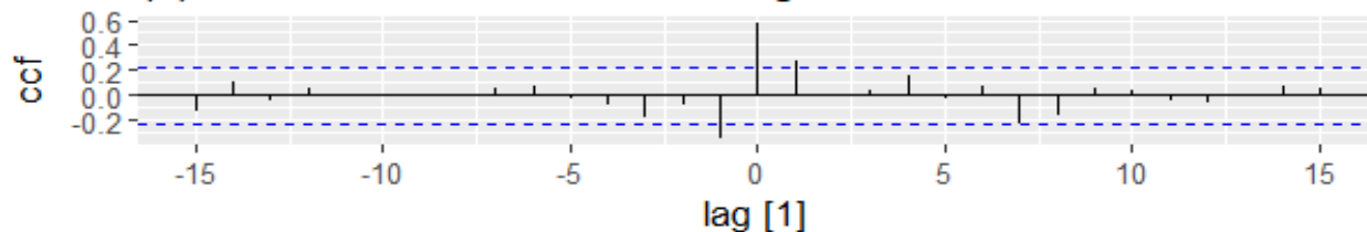
(d) 'Corona' with 'Distance education'
